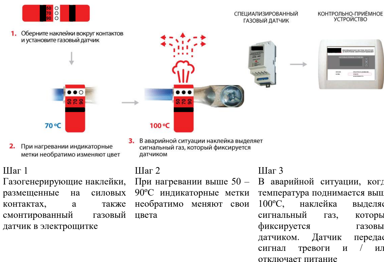
Рисунок 17. Пошаговая схема работы системы непрерывного контроля температуры на основе термоактивируемой газовыделяющей наклейки и специализированного газового датчика
